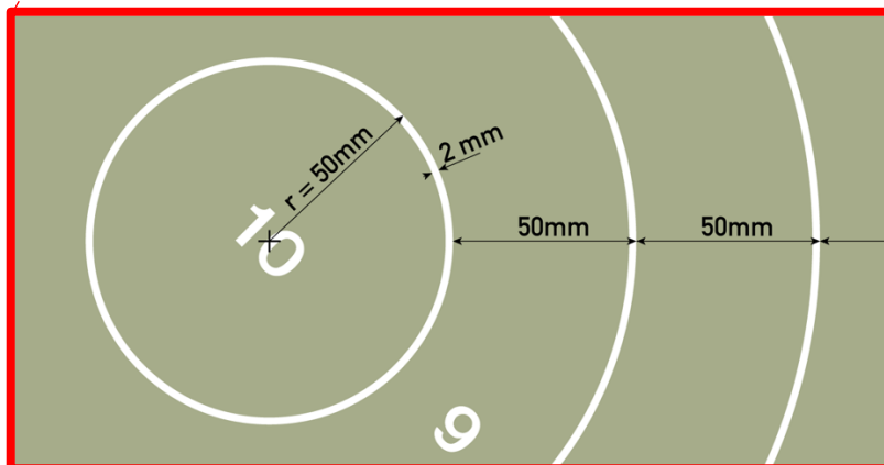
Obrázok 2: Detail s rozmermi
